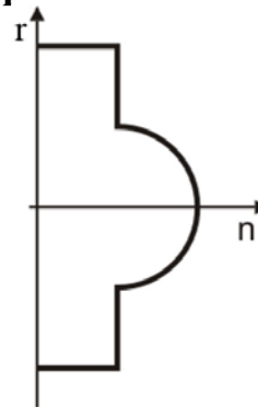
Mnohovidové optické vlákno s gradientní změnou indexu lomu
