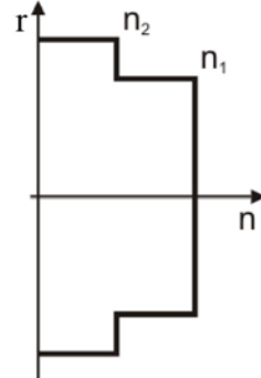
Mnohovidové optické vlákno se skokovou změnou indexu lomu
